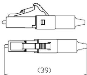
Sestavený konektor LC
