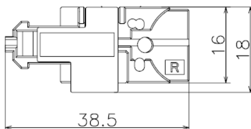
Rozměry držáku
